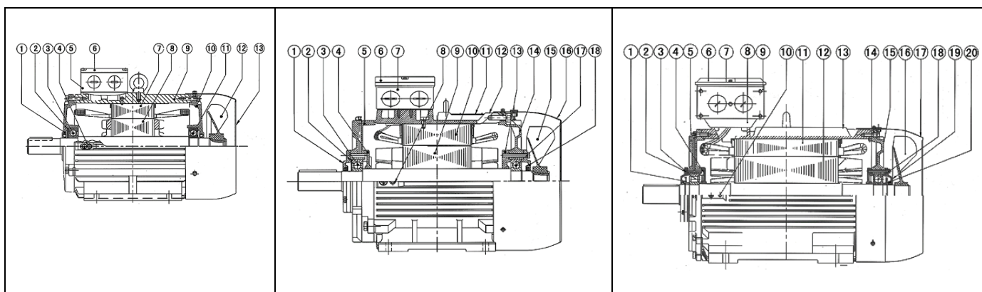
Motoren Achsenhöhe 80 – 132
